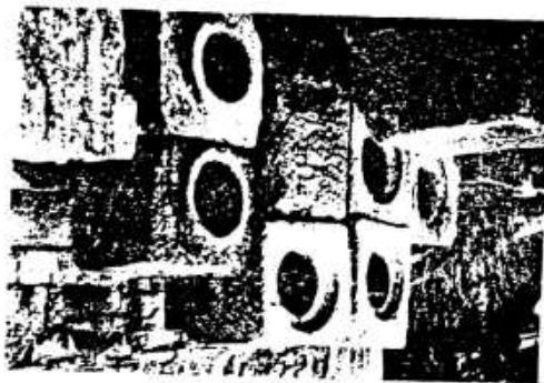
6. Efeso: blocchi provenienti da una condotta forzata in pietra, accatastati nell'agorà; alcuni (ad esempio in alto e al centro) presento lateralmente, un foro di ventilazione.
