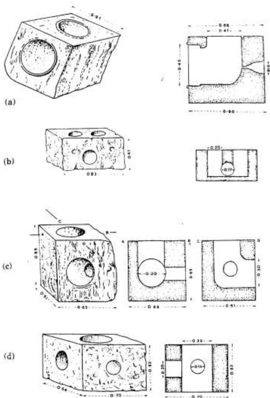
8. (a) Laodicea : blocco angolare proveniente da una condotta in pietra che illustra (in sezione) un probabile foro di ventilazione; (b) (c) (d) Smirne : vari blocchi angolari e di raccordo provenienti da tubature di un sifone in pietra (Weber)
