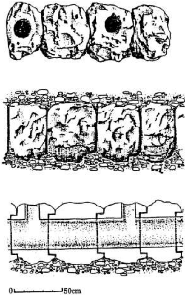
12. Hippos, Susa, Israele tubazioni di un sifone in pietra, in pianta, elevato e sezione, che mostrano fori (di ventilazione?) (Y. Peleg).
