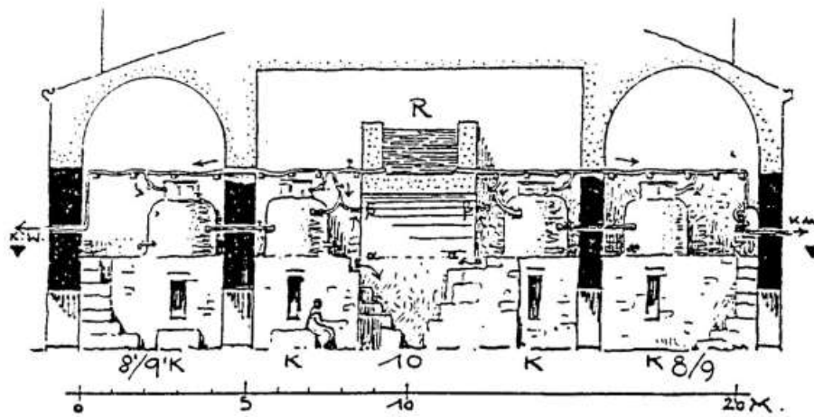
27. Lambesis : il locale delle caldaie nelle terme, con quattro caldaie (Krencker)
